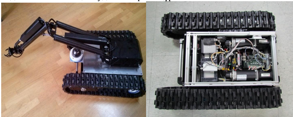
Сурет 7- Әскери және арнайы азаматтық қызметтерге арналған машиналық көру қабілетімен шынжыр табанды мобильді платформа.
