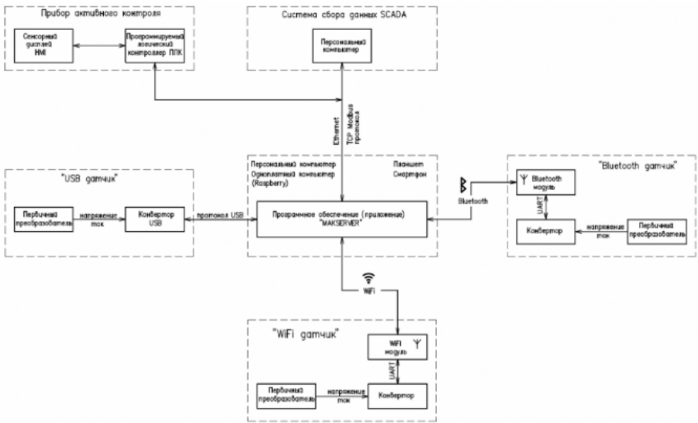
Рис. 2 - Состав и структура измерительных программно-аппаратных комплексов [28]
