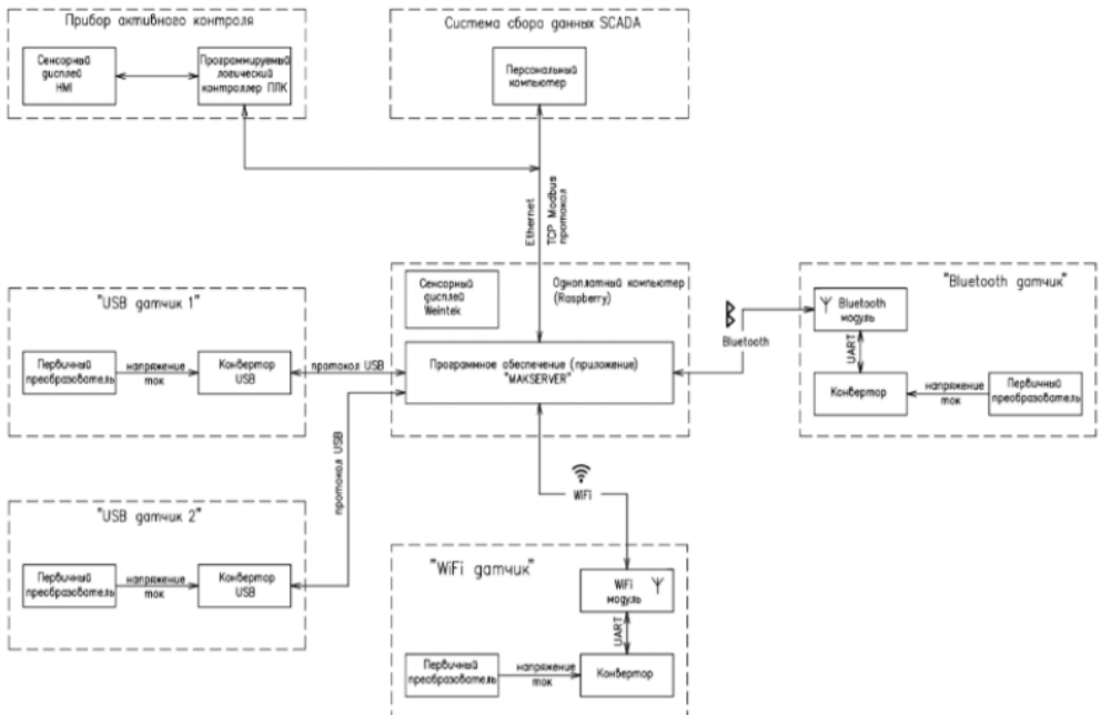
Рис. 3 - Структура блока индикации М-5.2 [28]
