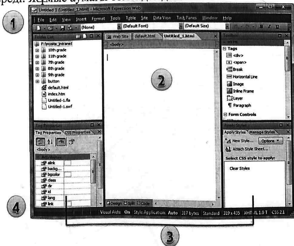
4-сурет. Expression Web бағдарламасының интерфейсі
